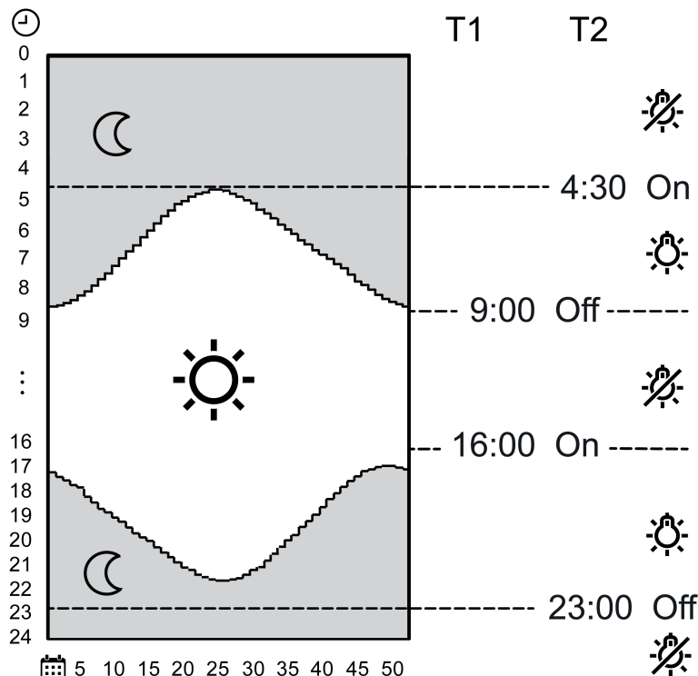
Рисунок 7: Пример использования зон памяти T1 и T2
