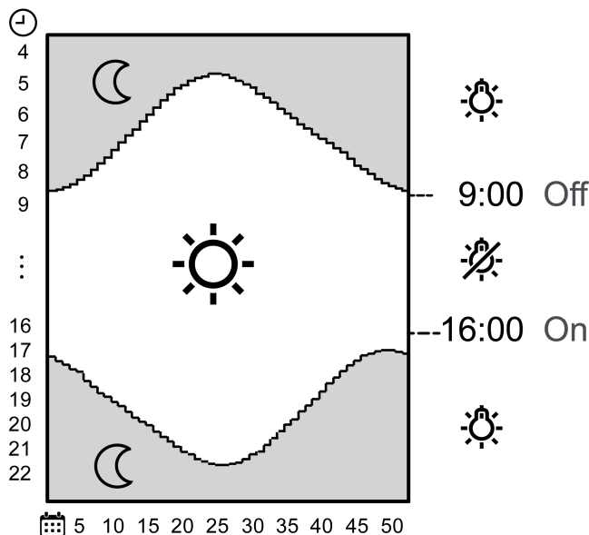
Рисунок 6: Заводские настройки: функция установки астрономического времени при использовании вставок для переключения и для выдержки времени
