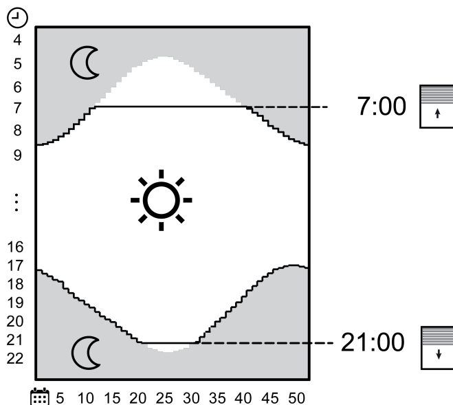
Рисунок 5: Заводские настройки: функция установки астрономического времени для вставок жалюзи
