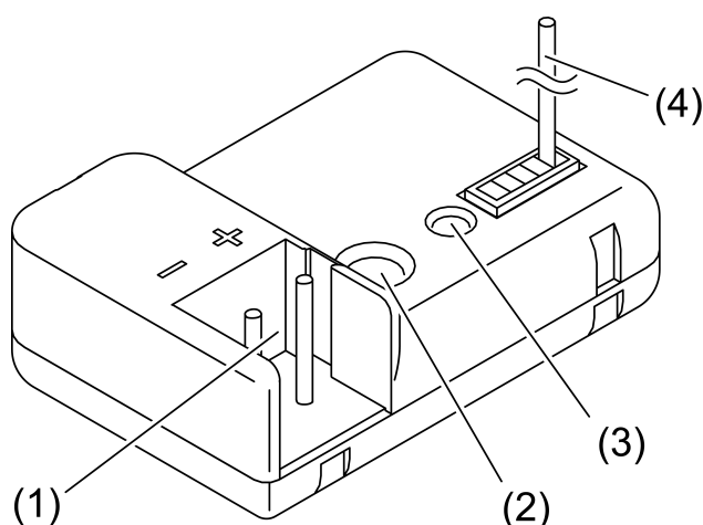
рисунок 1: Конструкция прибора
